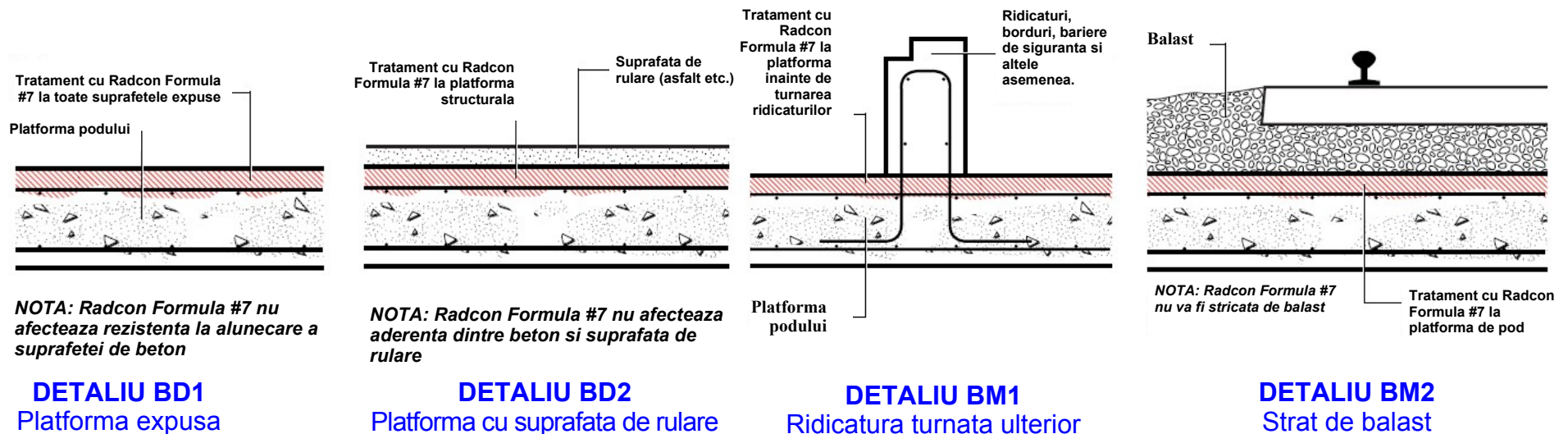
SECTIUNE TIPICA PRINTR-UN POD RUTIER
