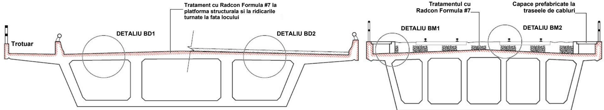
SECTIUNE TIPICA PRINTR-UN POD FERROVIAR
