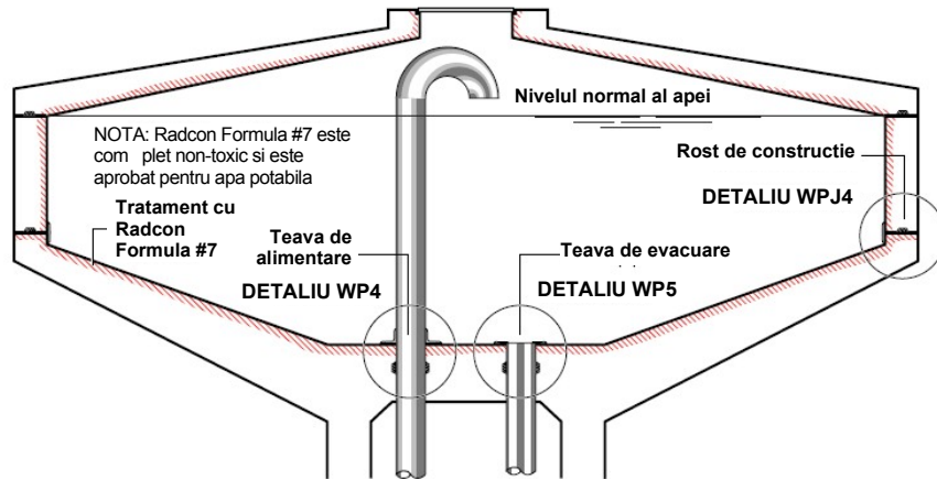
SECTIUNE TIPICA PRINTR-UN TURN DE APA SUSPENDAT
