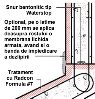
DETALIU WPJ4 Rost de constructie
