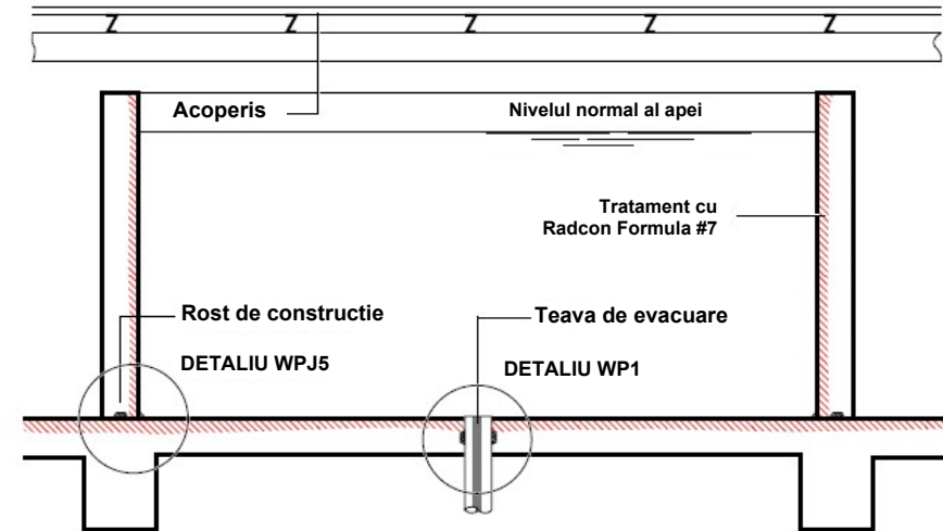
SECTIUNE TIPICA PRINTR-UN TURN DE APA, tip SPRINKLER
