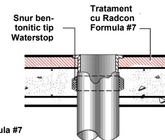
DETALIU WP1 Strapungere
