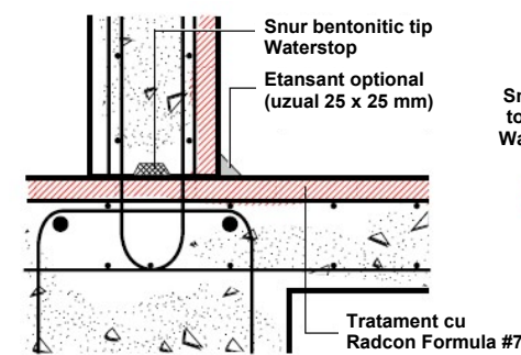
DETALIU WPJ6 Rost de constructie
