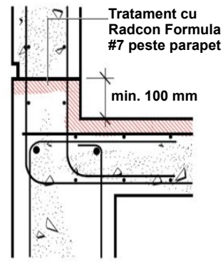
DETALIU PPJ2 Rost de constructie
