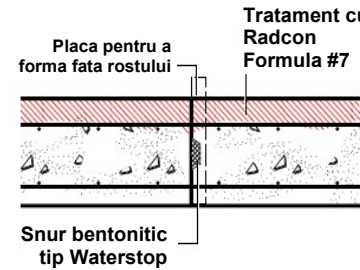
DETALIU PPJ1 Rost de constructie
