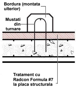
DETALIU PM1 Bordura
