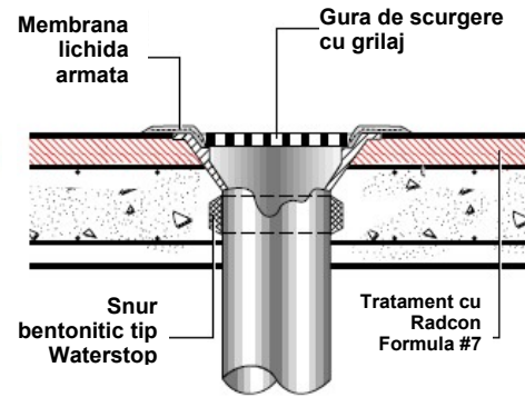
DETALIU PP3 Strapungere
